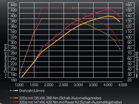
Leistungswerte des BMW 320d mit BMW Performance Power Kit Vollast 320d
